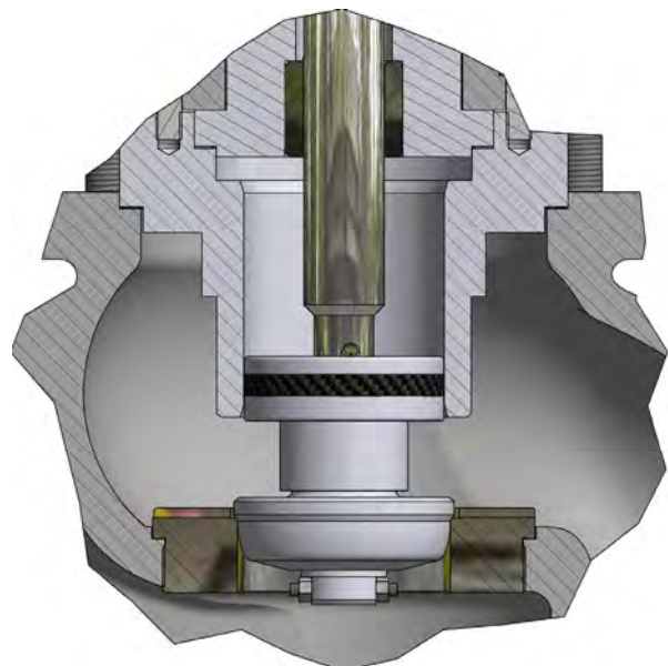
Otturatore bilanciato
