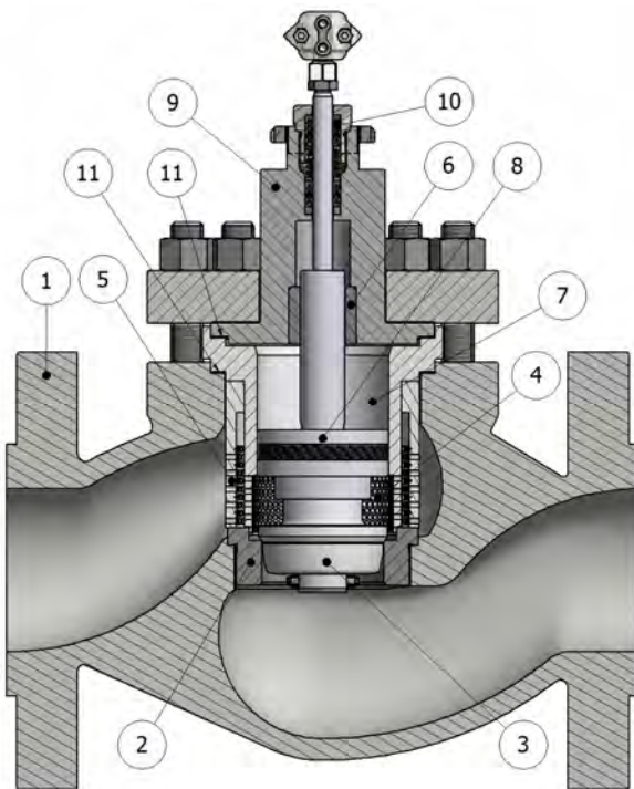
VALVOLA BILANCIATA CON DOPPIA GABBIA
