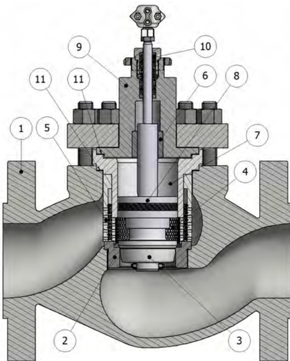
VALVOLA BILANCIATA
