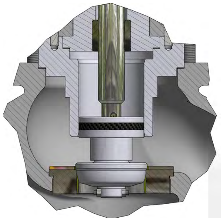
OTTURATORE BILANCIATO
